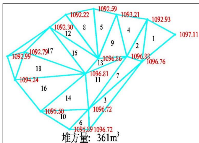
图4-3 SJ1工业场地内一分期设计“渣堆3”方量三角网法计算图
