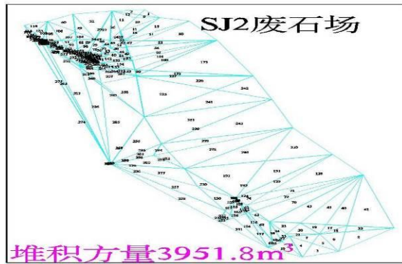
图 4-9 SJ2 废石场三角网法计算方量成果图
