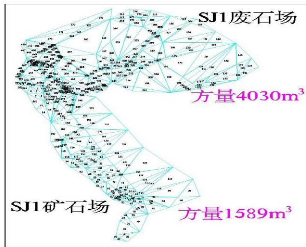
图4-4 SJ1废石场、SJ1矿石场三角网法土石方量计算图
