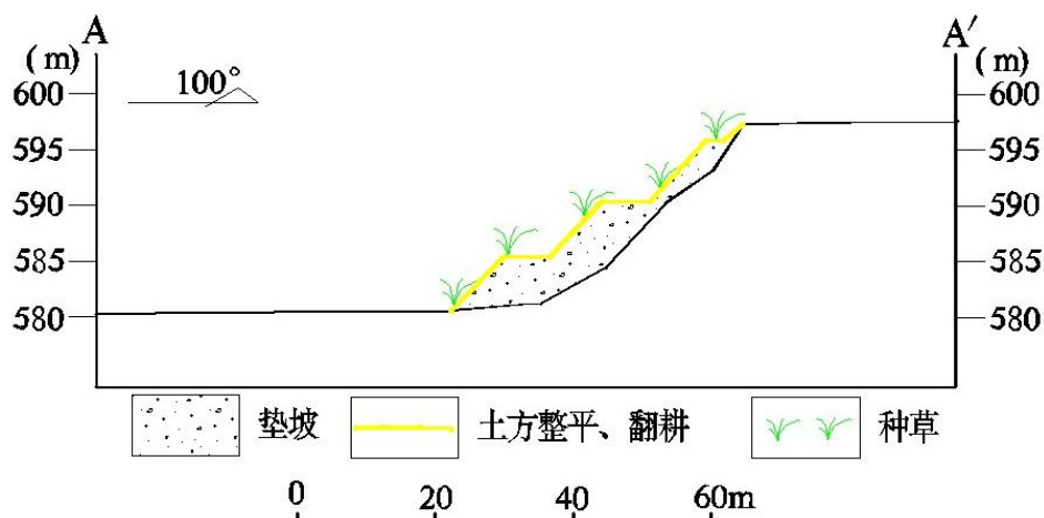
图 5-1 治理区西侧治理效果图
