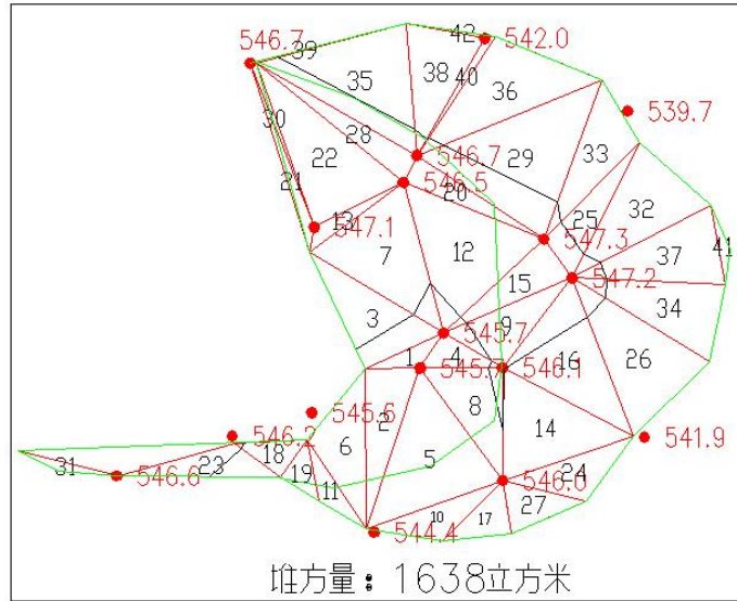
图4-7 FZ2废渣堆放方量三角网法计算成果图
