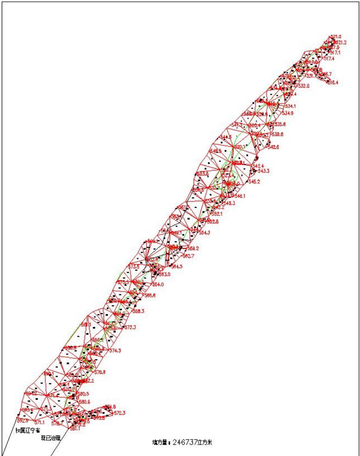
图 4-4 TK6 体积三角网法计算成果图
