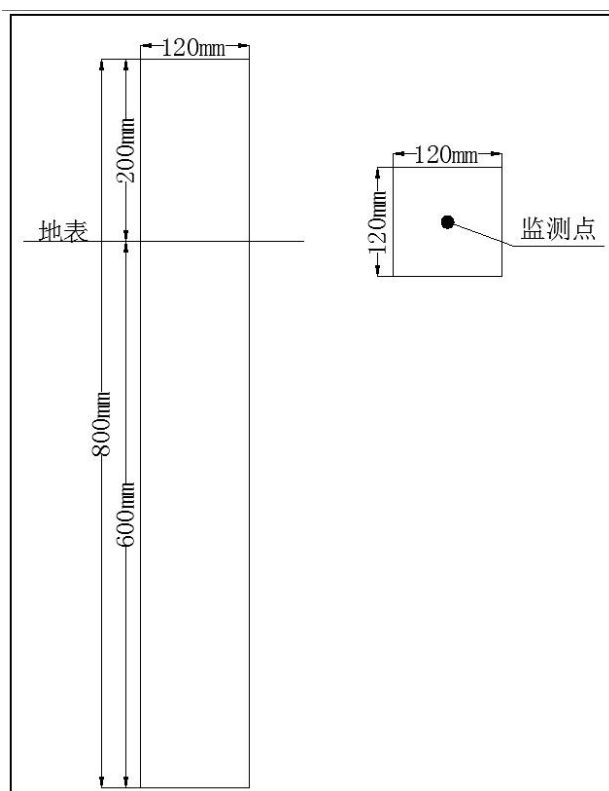
图 5-3 监测标桩示意图
