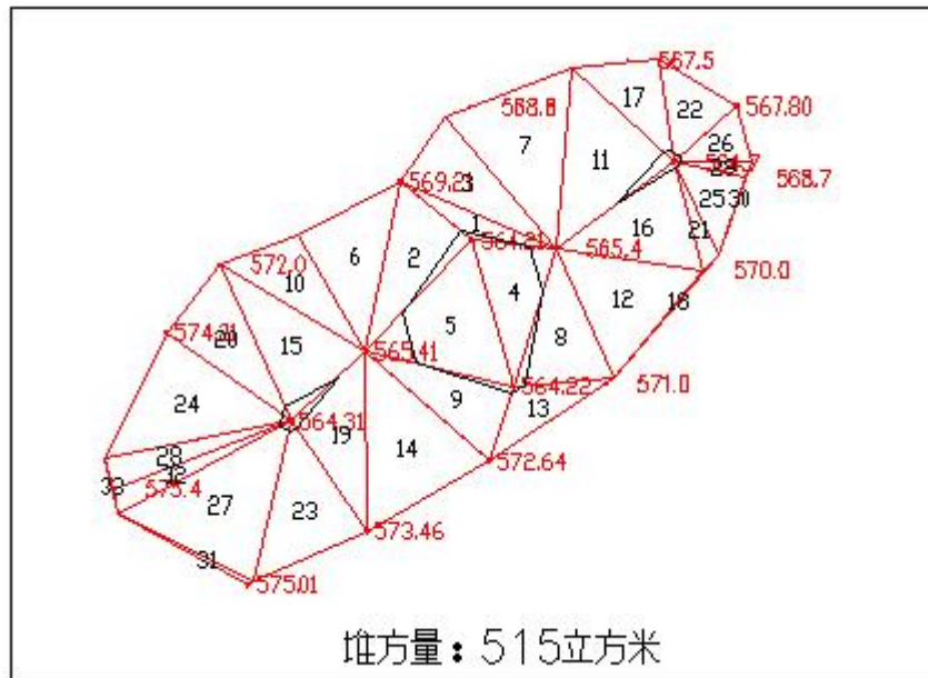
图4-2 TK4体积三角网法计算成果图
