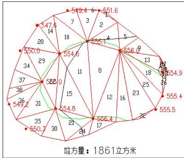
图4-8 FZ3废渣堆放方量三角网法计算成果图
