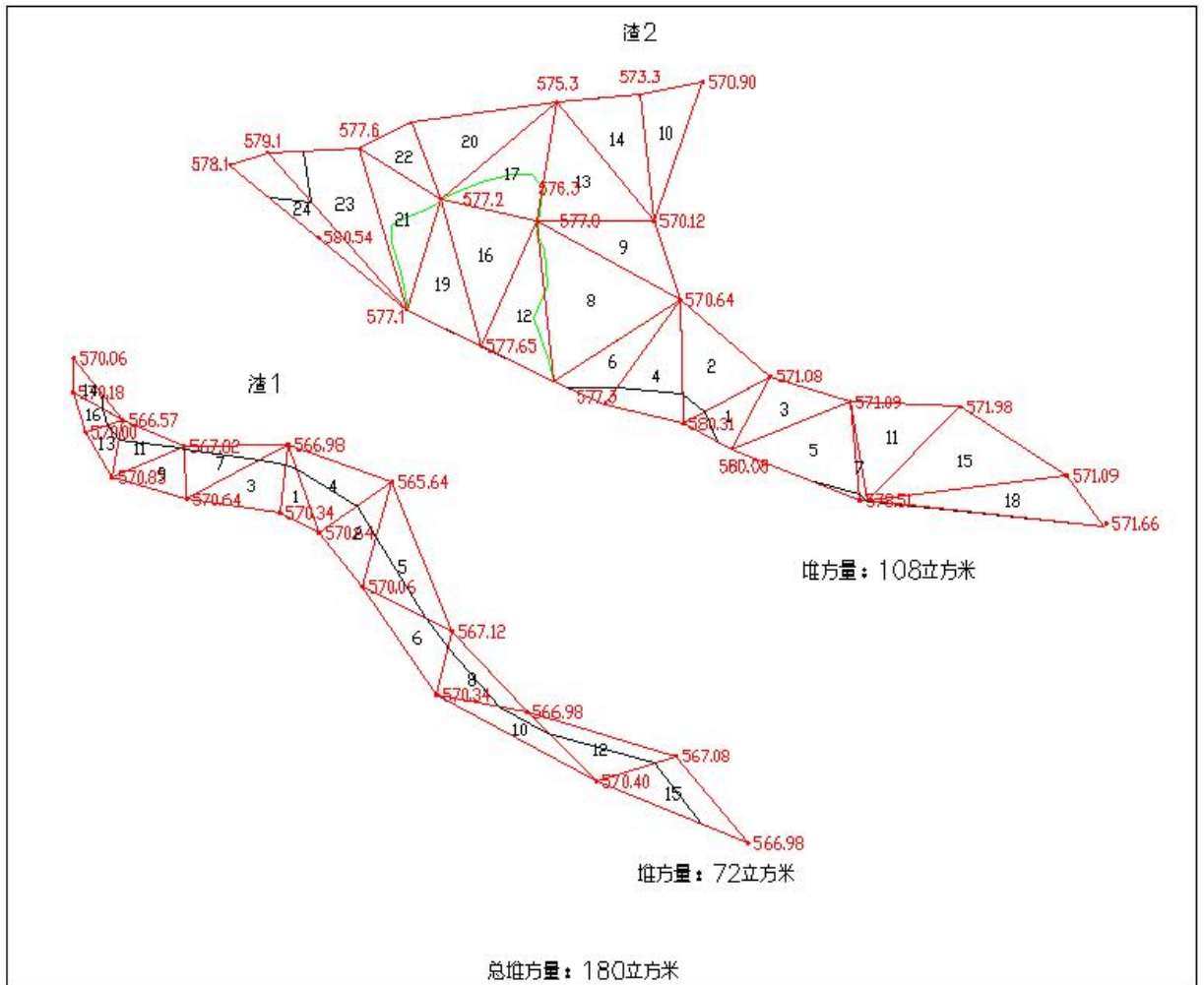
图4-10 FZ5废渣堆放方量三角网法计算成果图
