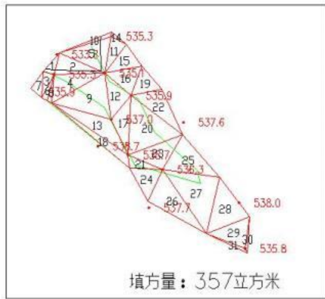
图3-5 TK7体积三角网法计算成果图
