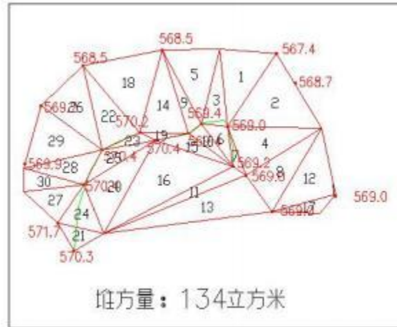
图3-12 表土堆2表土堆放方量三角网法计算成果图
