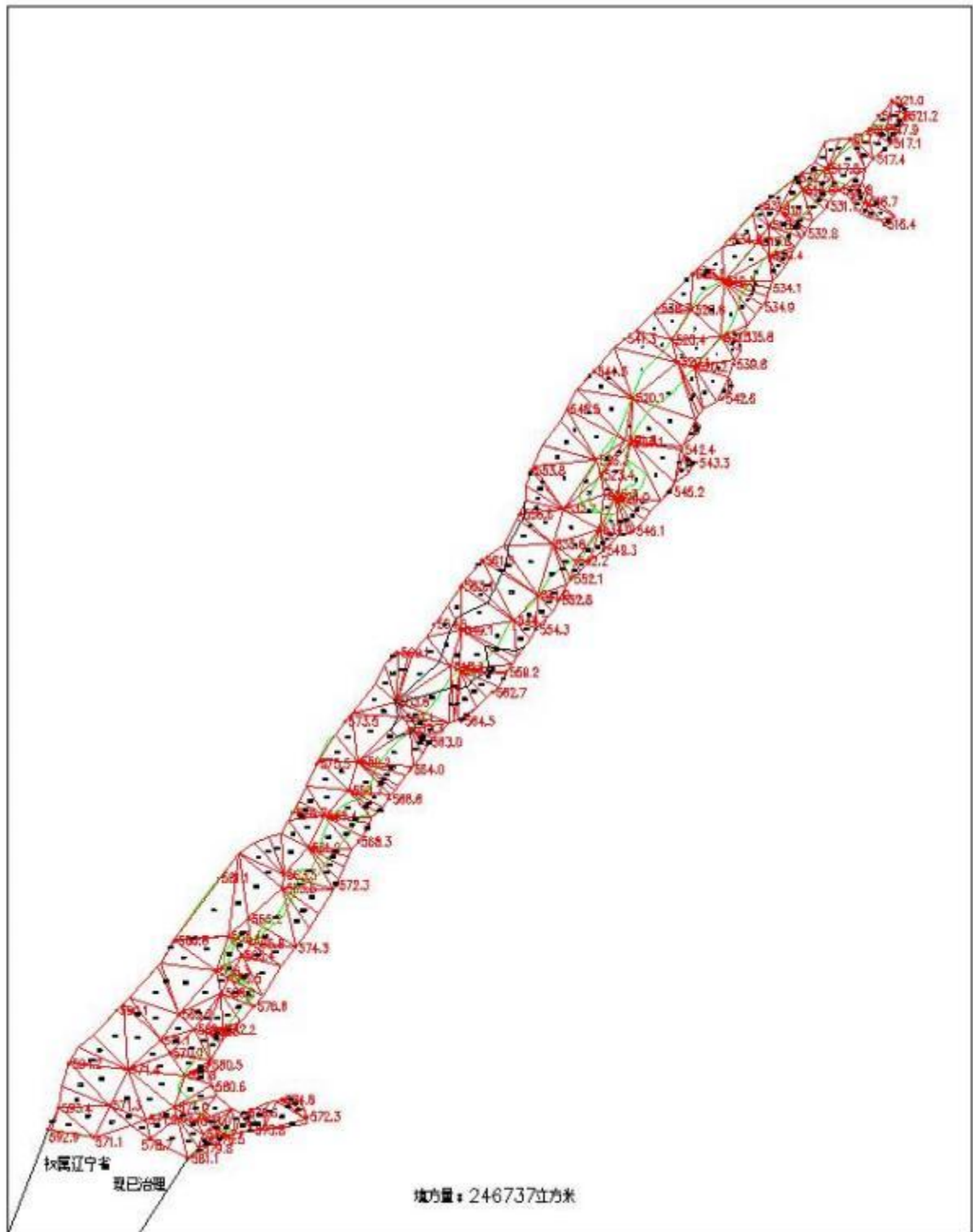
图 3-4 TK6 体积三角网法计算成果图
