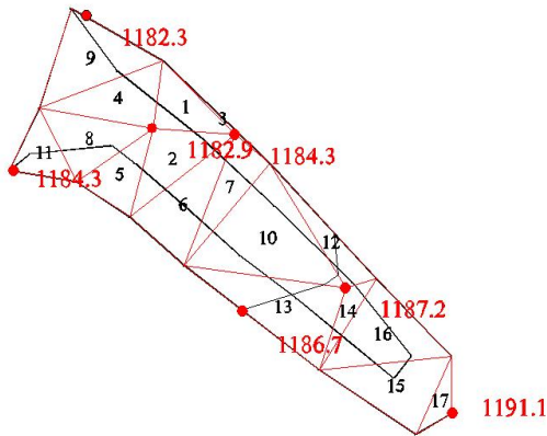
图 3-1 三角网法计算 PD2 挖方量成果图
