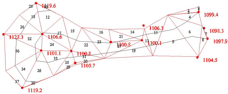
图 3-3 三角网法计算 PD5 挖方量成果图
