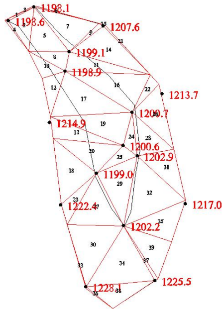
图 3-7 三角网法计算露天采坑 3 挖方量成果图
