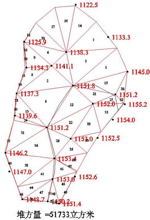
图3-11 三角网法计算3#废石堆堆方量成果图
