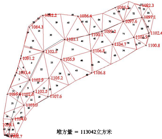
图 3-12 三角网法计算 4#废石堆堆方量成果图
