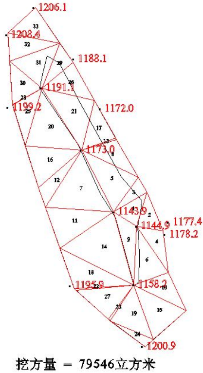
图3-5 三角网法计算露天采坑1挖方量成果图
