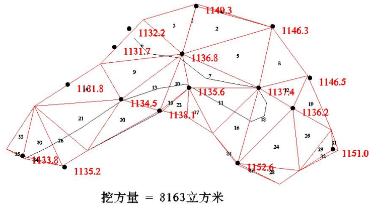
图 3-9 三角网法计算露天采坑 7 挖方量成果图
