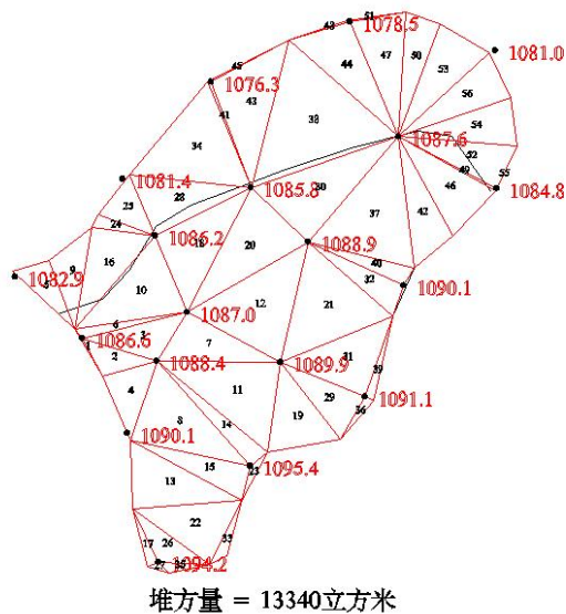
图3-13 三角网法计算5#废石堆堆方量成果图
