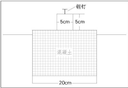
图 6-26 监测桩设计图
